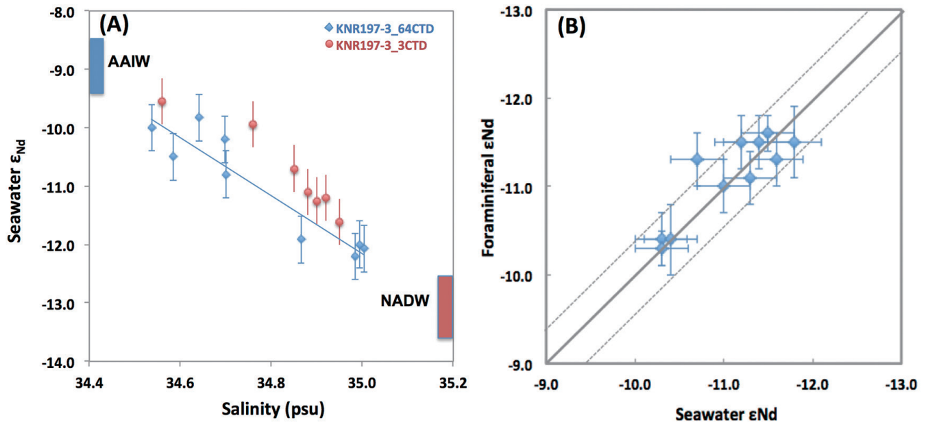
圖一(A) 海水釷同位素比值對鹽度作圖; (B) 海洋表層沈積物中有孔蟲殼體內鐵錳氧化物釷同位素比值與海水釷同位素的關係[2]。
