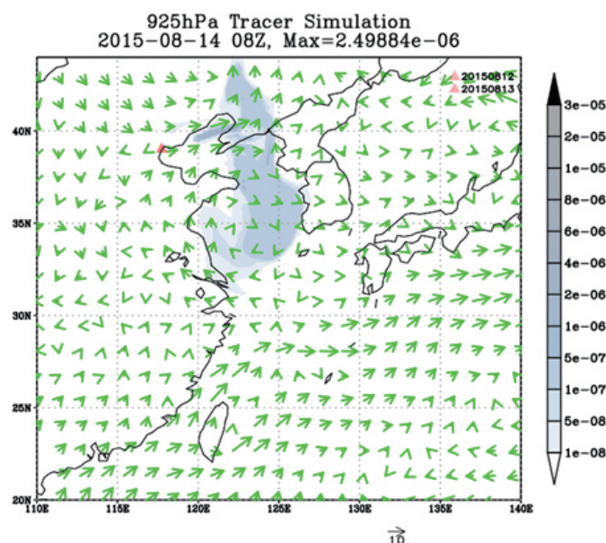
圖二 WRF/Chem 模式模擬天津港大爆炸事故後8月14日 16:00 LST，空氣汙染物在925 hPa等壓面的擴散情形
