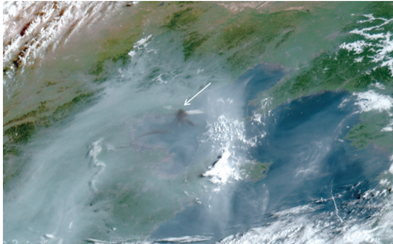
圖一 8月12日日本同步氣象衛星向日葵所拍攝之真色圖像，圖中白色箭頭所指之黑色團狀物，即為爆炸後產生之濃煙，與周遭日常灰白色空汙不同。（圖像為美國海洋大氣總署Dr. Dan Lindsey提供）
