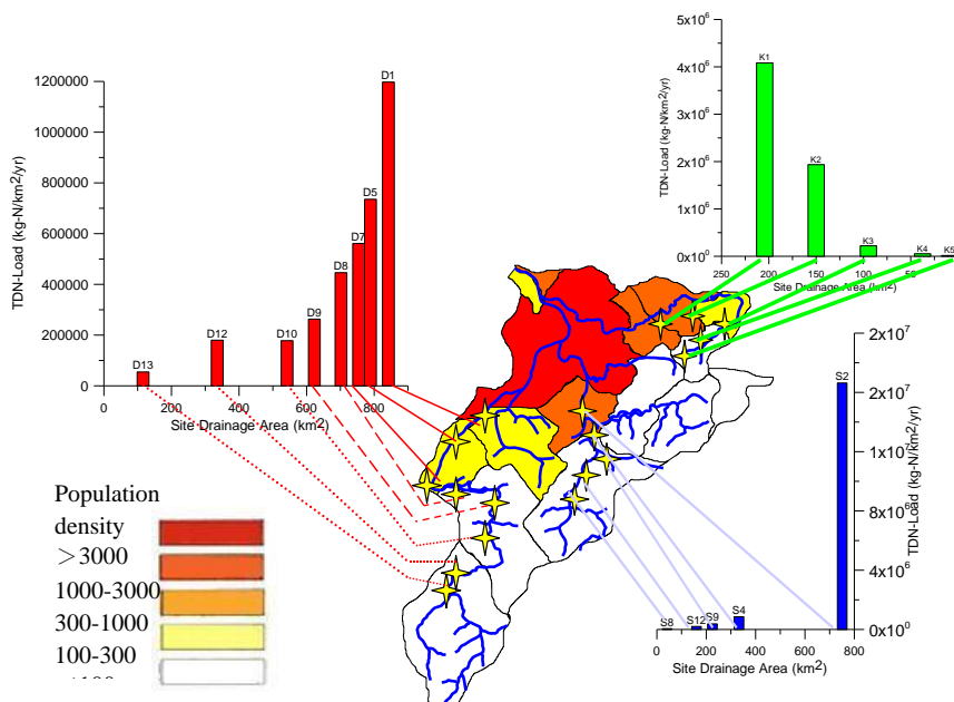
圖 2. 總氮(Total Nitrogen)單位面積產值空間分佈圖(單位為 \text{Kg-N/km}^2/\text{y} )。
