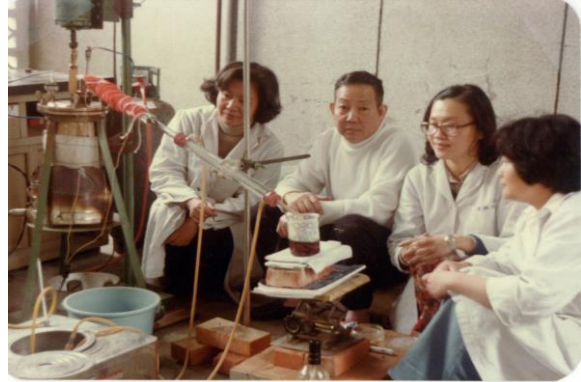
民國 67 年冬，利用特別設計製作之蒸餾裝置，以分餾煤焦油中之化學成分。分餾煤焦油時氣味難聞，但當時實驗室裡缺少抽氣櫥設備，只好將整套裝置擺在走廊盡頭通風處。冬冷夏熱、偶而還會遭雨淋，克難地進行研究。
